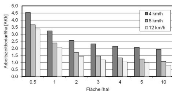
Abb. 8: Vergleich des Arbeitszeitbedarfs kameragesteuerter Hackgeräte mit 3m Arbeitsbreite bei unterschiedlichen Arbeitsgeschwindigkeiten.
